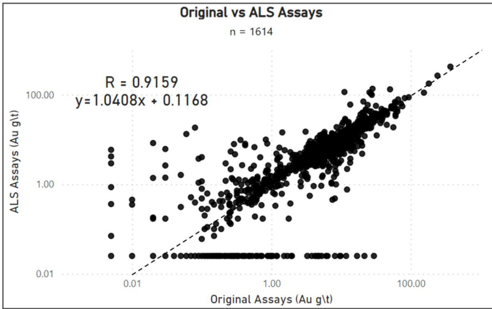
Figure STYLEREF 1 \s 8-. Mine Laboratory Pulp External Check Assays at ALS (2021-2023)
